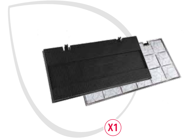
KFC6911 (CP150) 35602054 EAN 8016361971271 435x217x20mm; 1110gr - Typ 150
