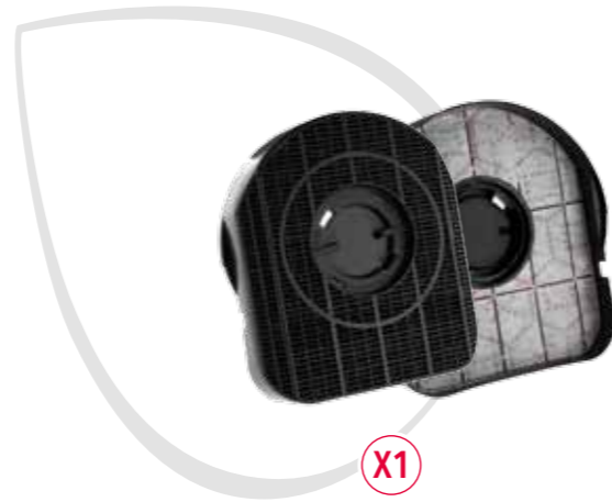
KFC6920 (CP200) 35602063 EAN 8016361972964 208x180x48mm; 390gr - Typ 200
