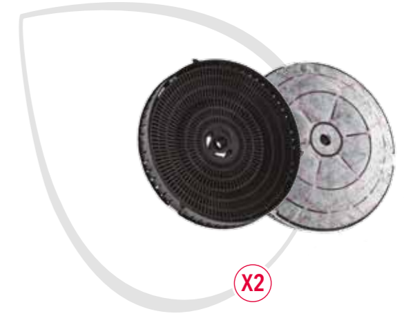
KFC6915 (CP057) 35602058 EAN 8016361971318 Ø175x45mm; 406gr - Typ 057 - 2 filtre v balení
